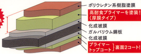
構造図
